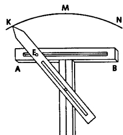
Mechanischer Apparat zur Erzeugung der Konchoide KMN. (E bewegt sich auf der Richtlinie AB, so daß der »Abstand« EK konstant ist).
